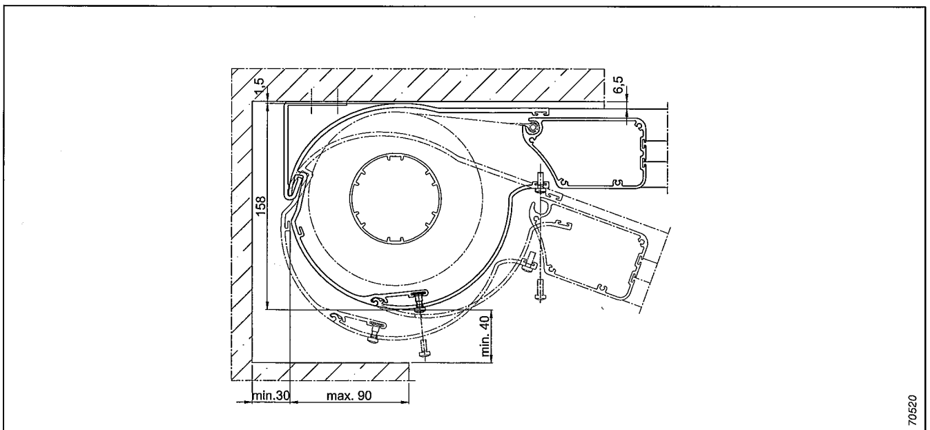
Abb. 327: Einbauraum Blende
